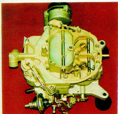
AUTOLITE 4300
