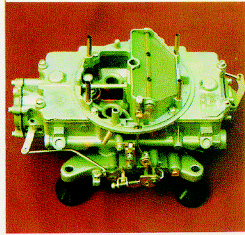
AUTOLITE 4100 "HI-PO"
