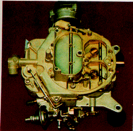
AUTOLITE 4300
