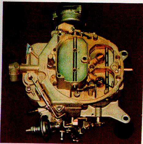
AUTOLITE 4300
