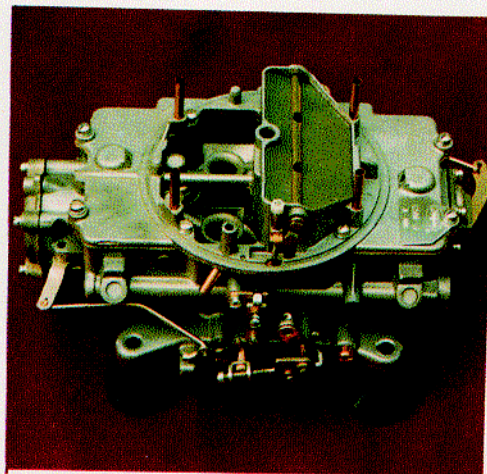
AUTOLITE 4100 "HI-PO"
