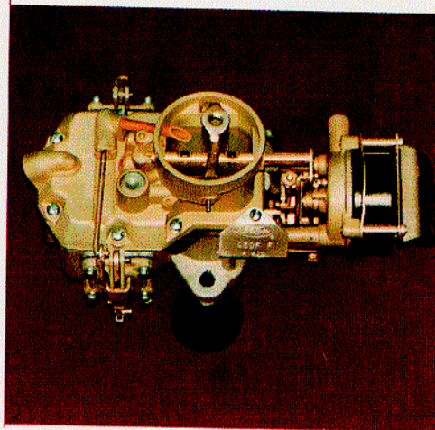
AUTOLITE 1100
