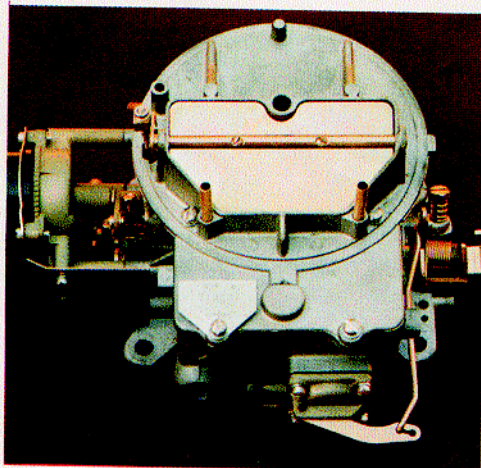
AUTOLITE 2100
