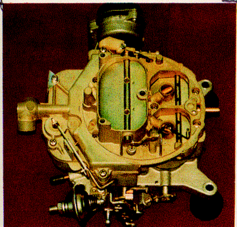
AUTOLITE 4300
