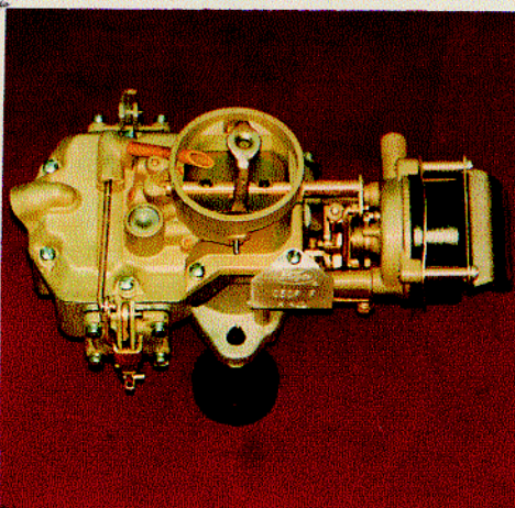
AUTOLITE 1100
