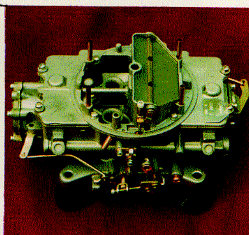
AUTOLITE 4100 "HI-PO"
