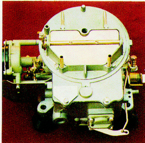
AUTOLITE 2100
