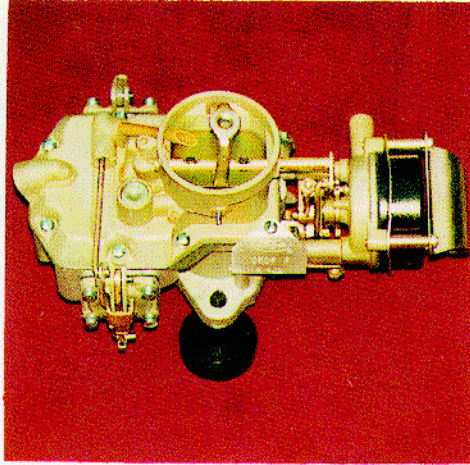
AUTOLITE 1100
