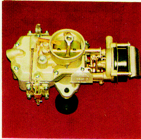
AUTOLITE 1100
