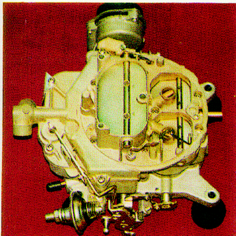
AUTOLITE 4300
