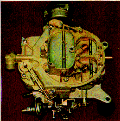
AUTOLITE 4300
