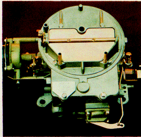
AUTOLITE 2100
