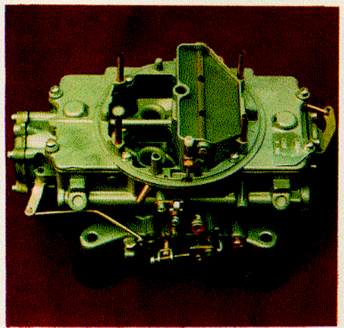
AUTOLITE 4100 "HI-PO"
