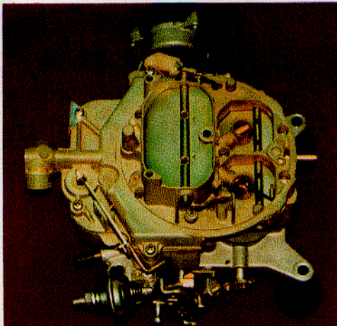
AUTOLITE 4300
