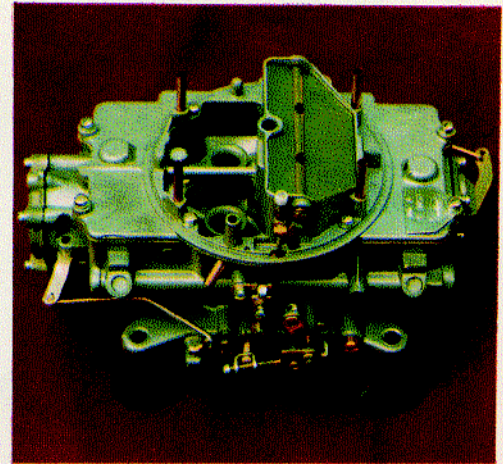
AUTOLITE 4100 "HI-PO"
