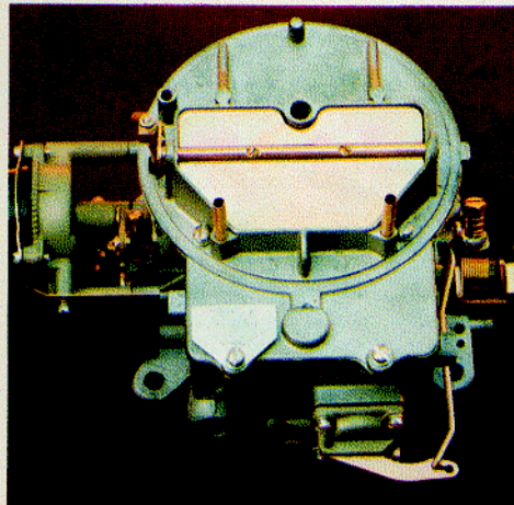
AUTOLITE 2100
