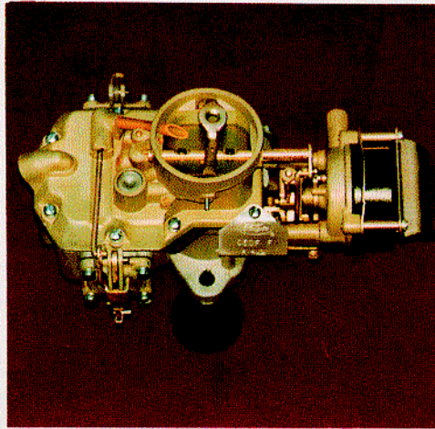
AUTOLITE 1100
