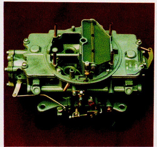
AUTOLITE 4100 "HI-PO"
