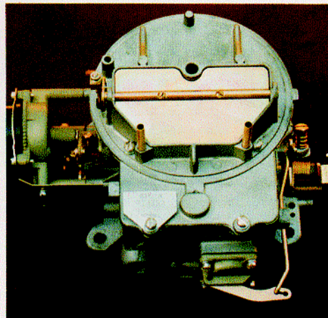
AUTOLITE 2100
