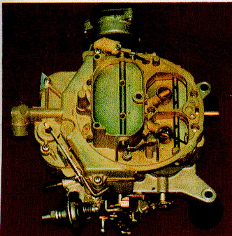
AUTOLITE 4300
