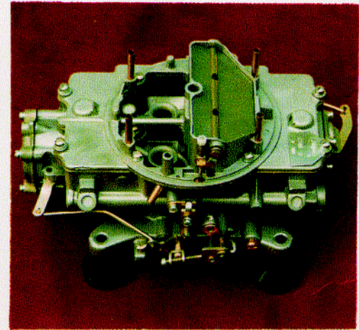
AUTOLITE 4100 "HI-PO"
