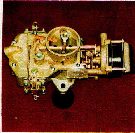
AUTOLITE 1100
